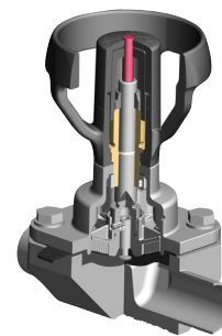
Schnittbild SISTO-C 2/2 Membranventil mit neuer Oberteilgeneration
